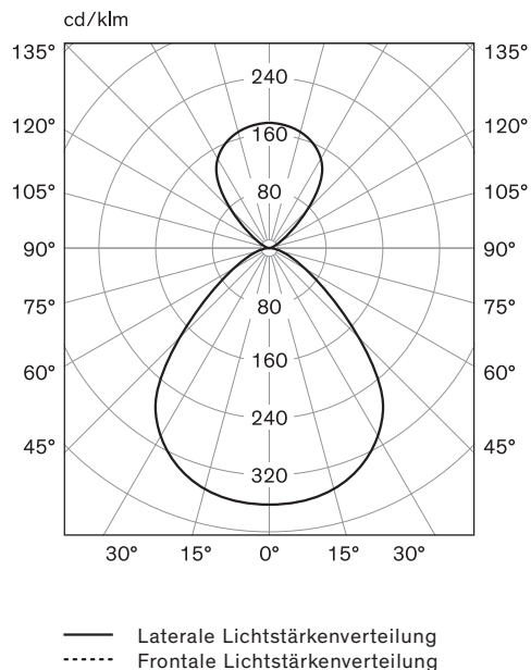
Lichtstärkenverteilung
