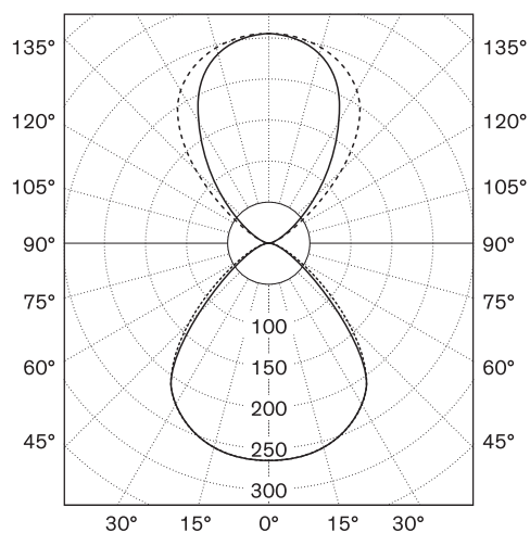
Lichtstärkenverteilung cd/klm
