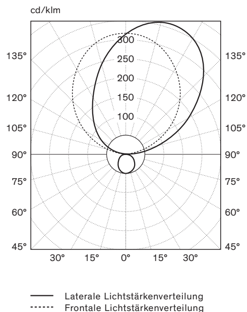
Lichtstärkenverteilung
