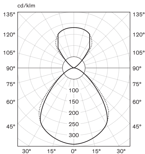
Lichtstärkenverteilung
